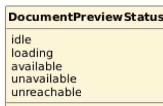
Figura 106: Tipo — DocumentPreviewStatus
