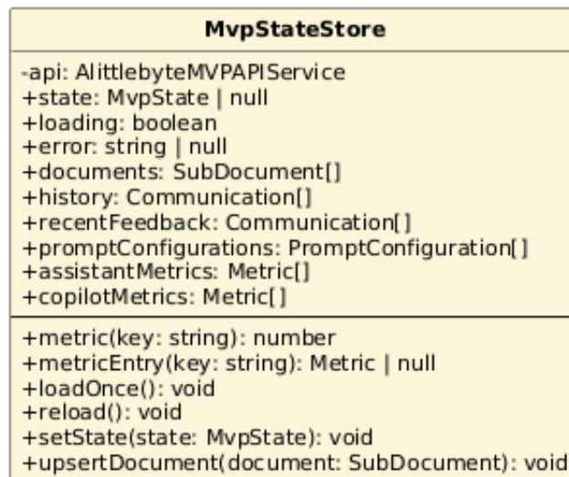
Figura 92: Classe — MvpStateStore
