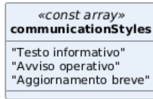
Figura 99: Tipo — communicationStyles
