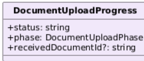
Figura 104: Tipo — DocumentUploadProgress
