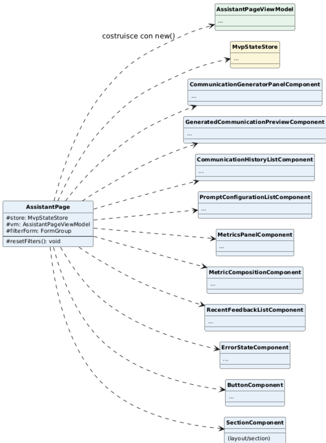
Figura 122: Classe — AssistantPage
