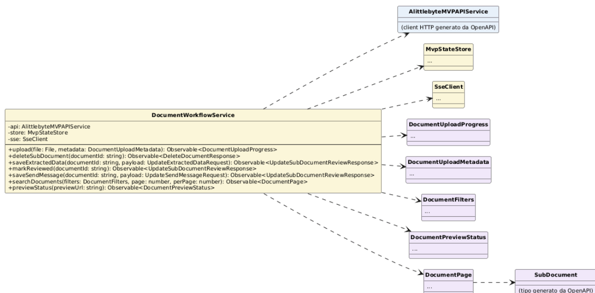
Figura 109: Classe — DocumentWorkflowService
