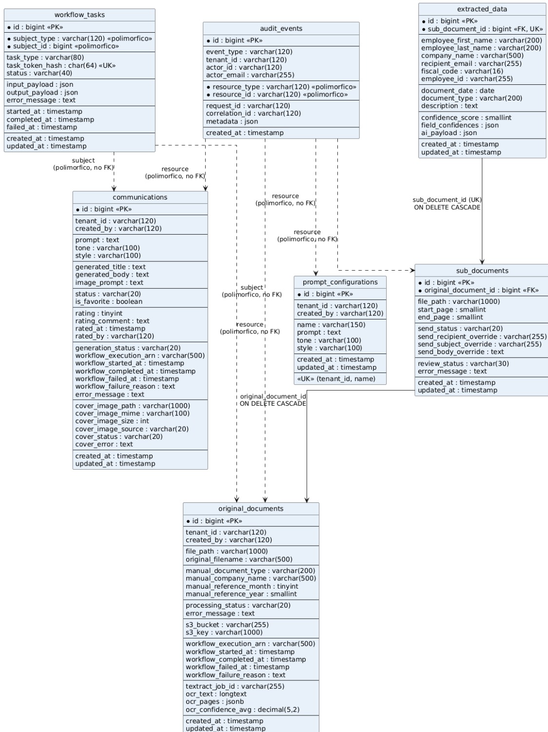
Figura 126: Schema Relazionale
